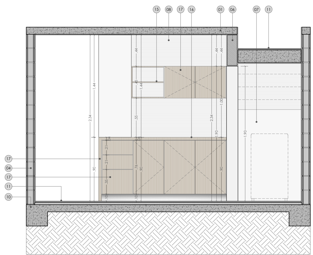
SECCIÓN 2 / ESC. 1:25
